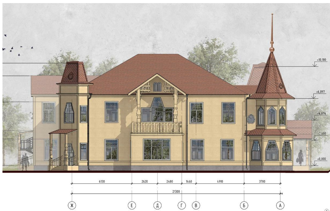
Фасад Ж-А
