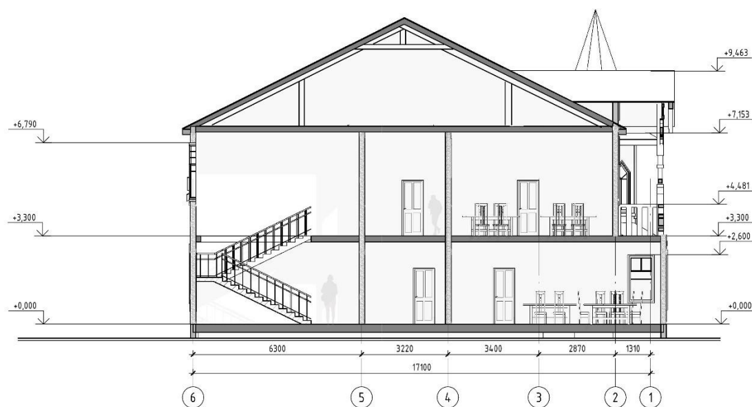
Разрез 1-1
