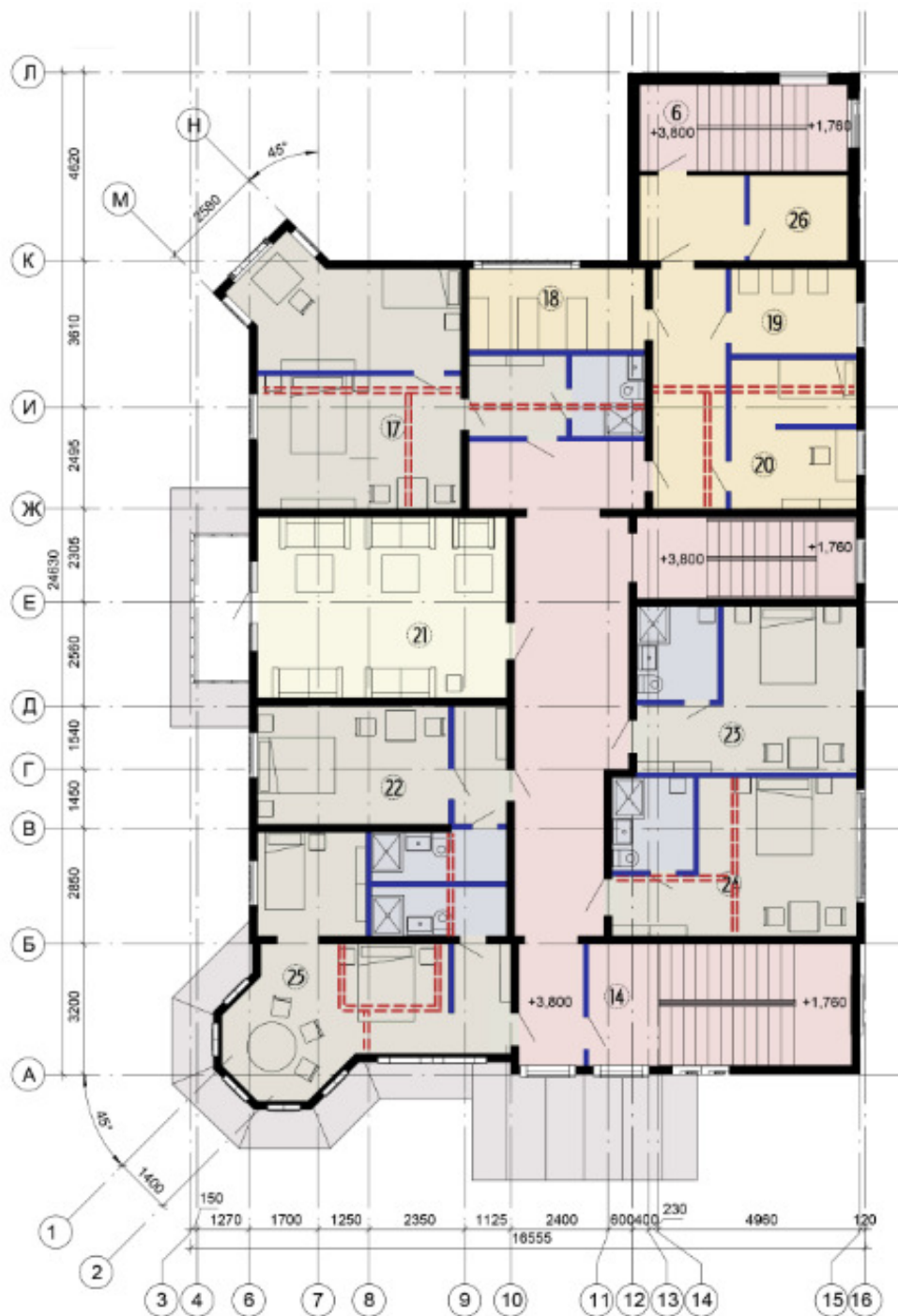
План 2 этажа
