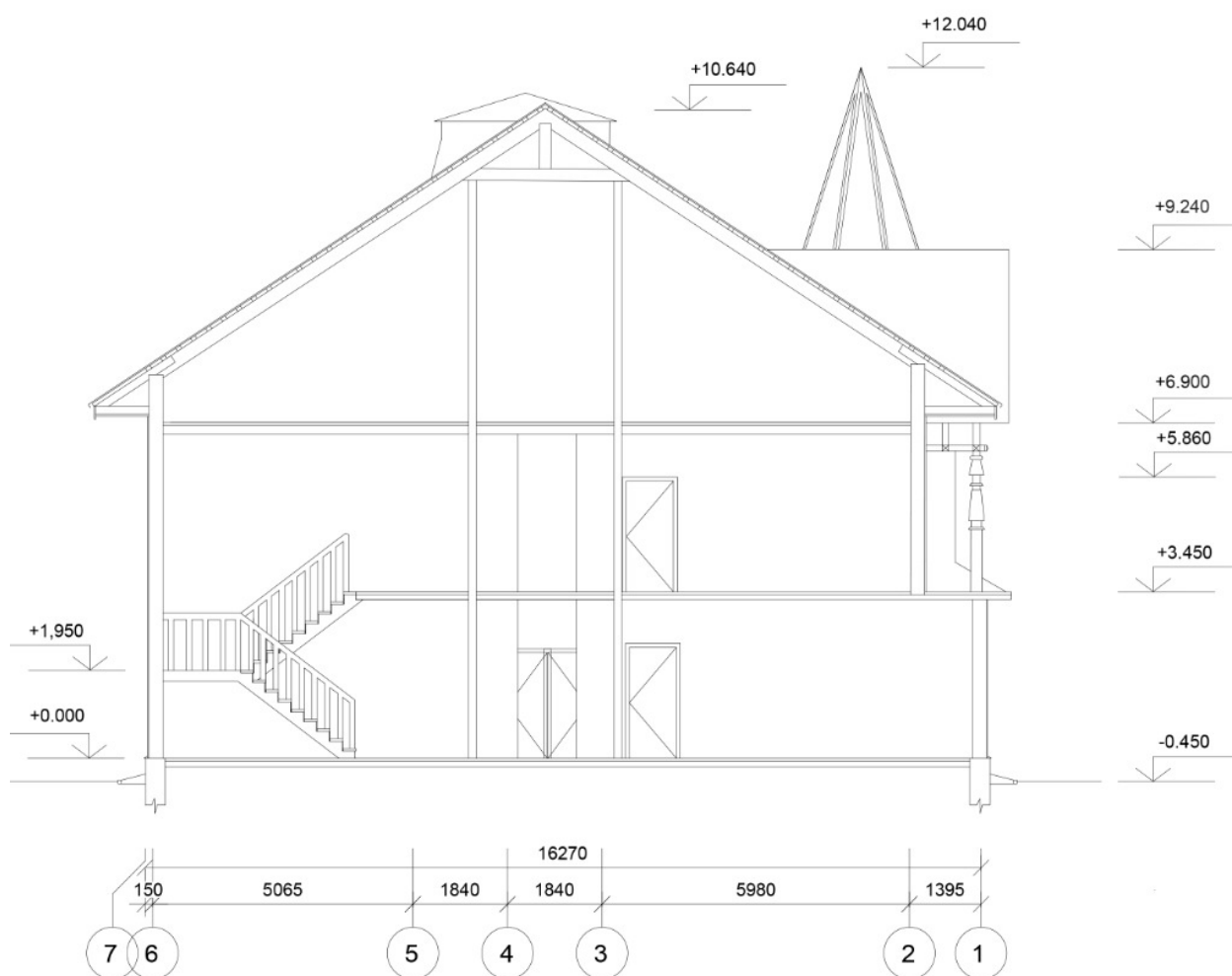
Разрез 1-1
