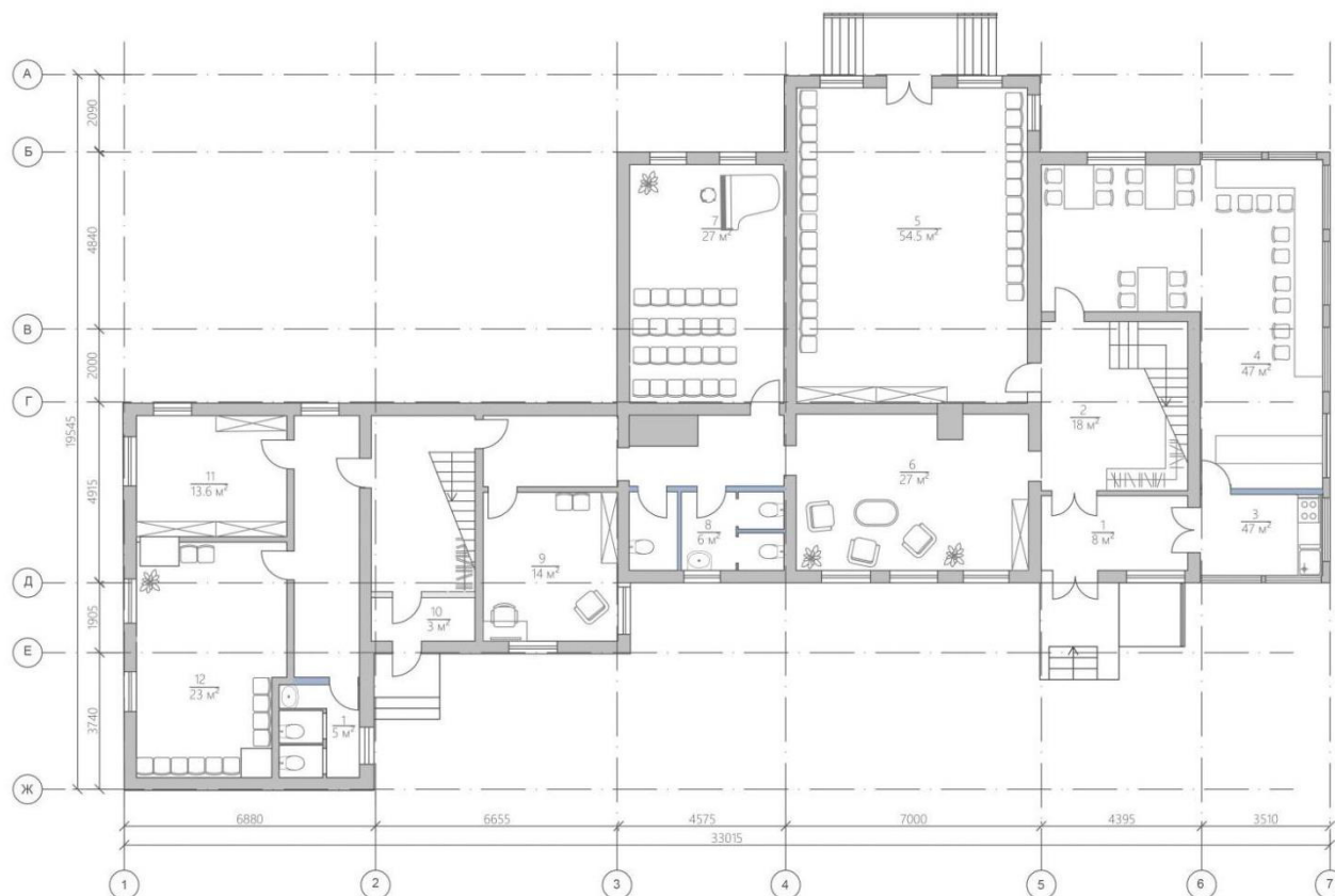
Экспликация 1 этажа
