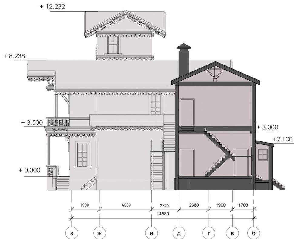
Разрез на осях 3-Б
