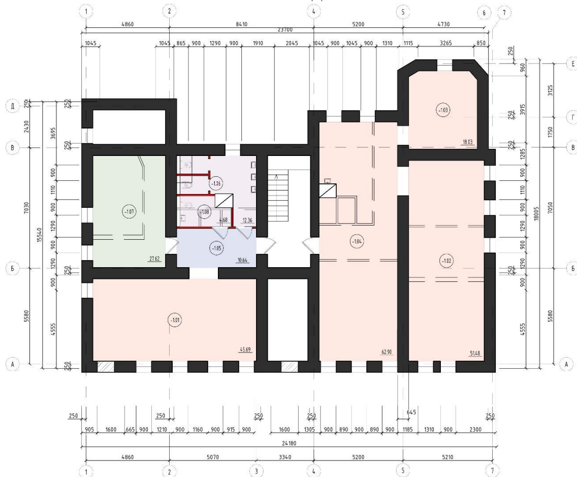
План подвала
