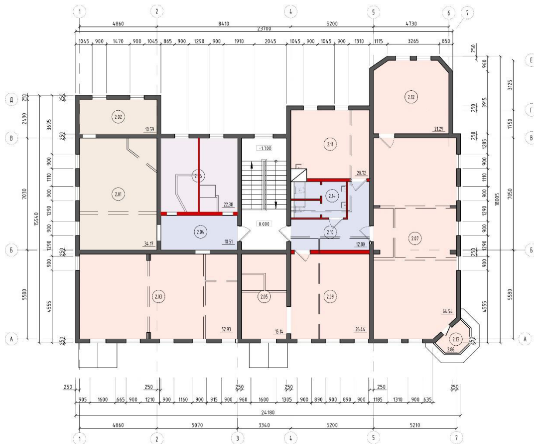
План 2 этажа
